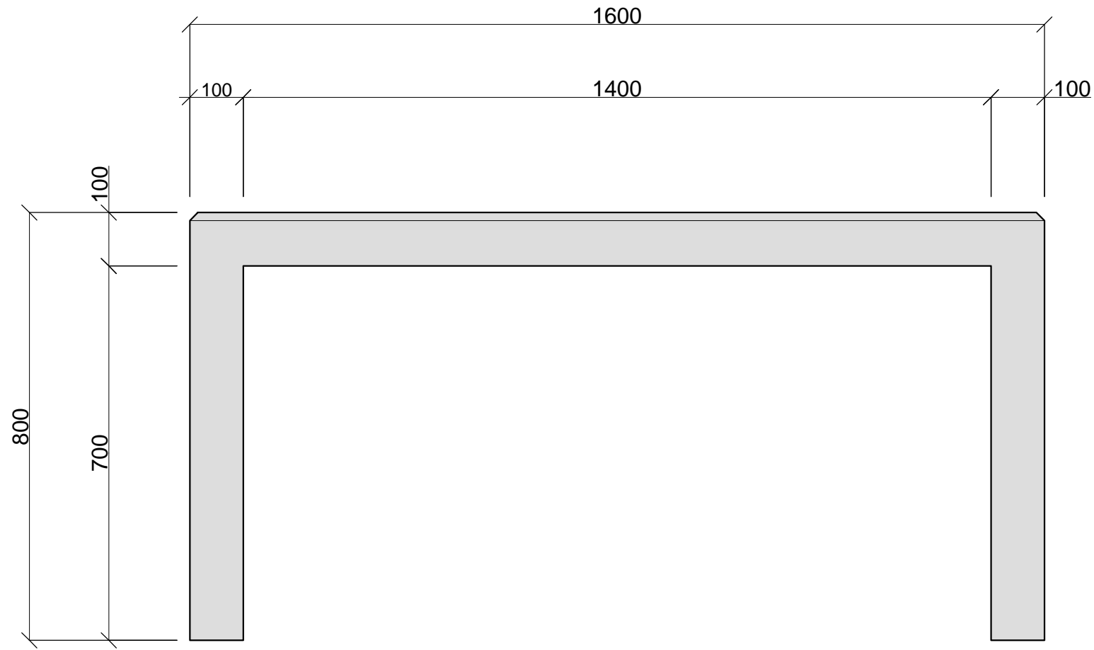
ELEVATION
